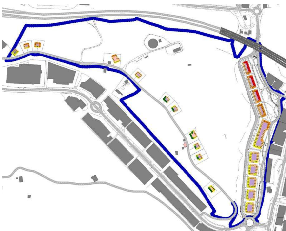
MAPA DE NIVELES SONOROS. MAPA DE FACHADAS. ESCENARIO: FUTURO PERIODO DE EVALUACIÓN: NOCHE
