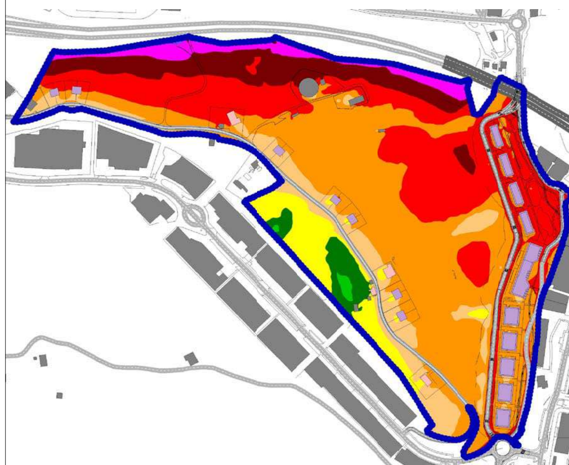
MAPA DE NIVELES SONOROS A 2 METROS DE ALTURA. ESCENARIO: FUTURO PERIODO DE EVALUACIÓN: TARDE
