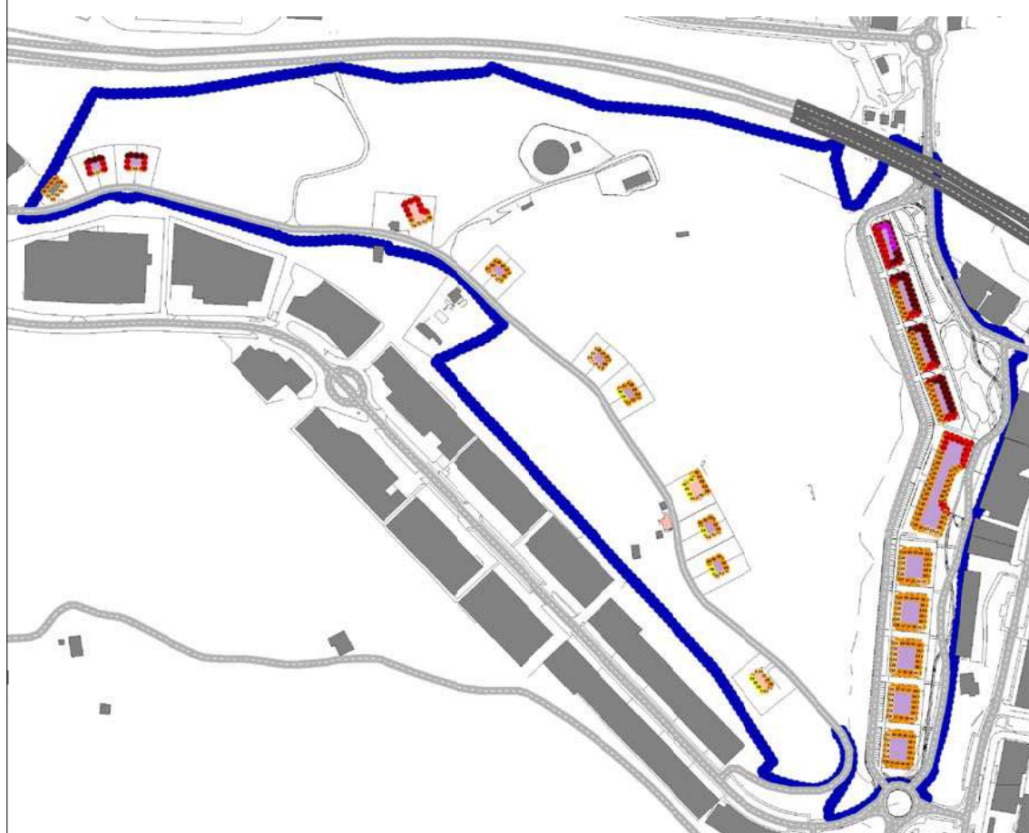
MAPA DE NIVELES SONOROS. MAPA DE FACHADAS. ESCENARIO: FUTURO PERIODO DE EVALUACIÓN: DIA
