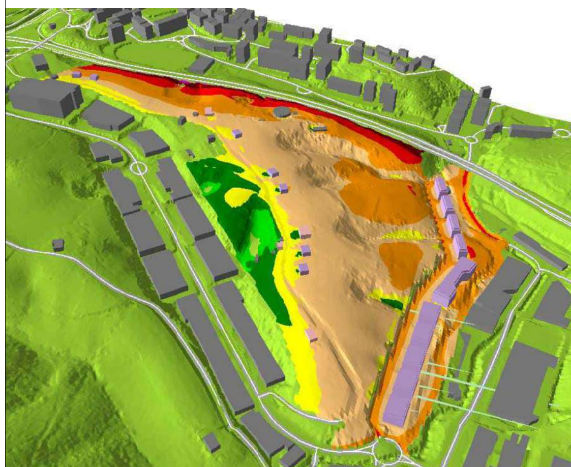
MAPA DE NIVELES SONOROS A 2 METROS DE ALTURA. ESCENARIO: FUTURO PERIODO DE EVALUACIÓN: IMAGEN 3D NOCHE
