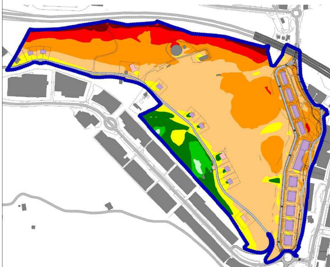
MAPA DE NIVELES SONOROS A 2 METROS DE ALTURA. ESCENARIO: FUTURO PERIODO DE EVALUACIÓN: NOCHE
