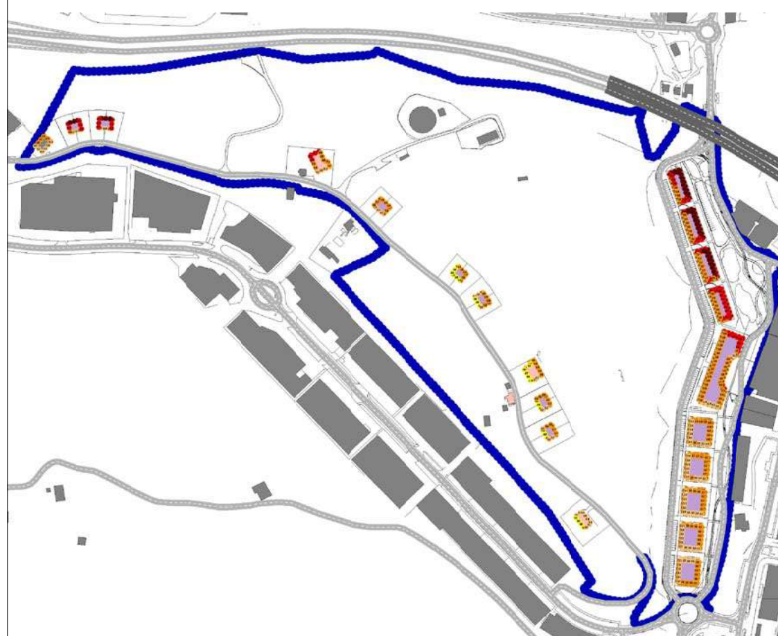
MAPA DE NIVELES SONOROS. MAPA DE FACHADAS. ESCENARIO: FUTURO PERIODO DE EVALUACIÓN: TARDE
