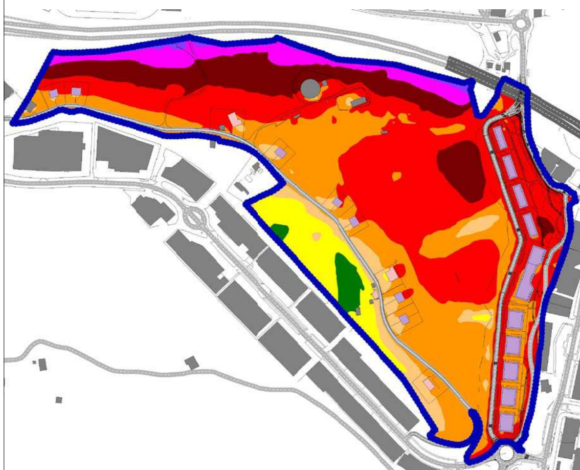
MAPA DE NIVELES SONOROS A 2 METROS DE ALTURA. ESCENARIO: FUTURO PERIODO DE EVALUACIÓN: DIA
