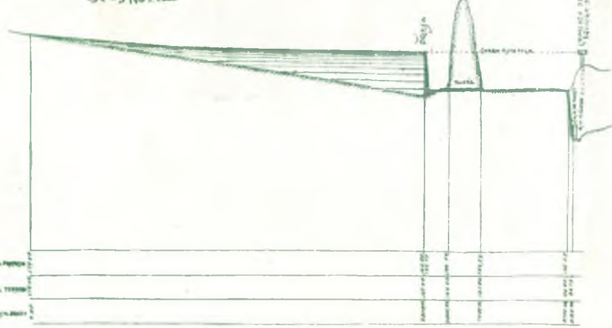
PERFIL LONGITUDINAL Escala de 1:2000
