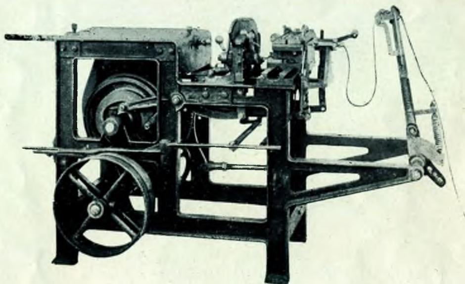
Cosedora lateral para suelas de alpargatas
