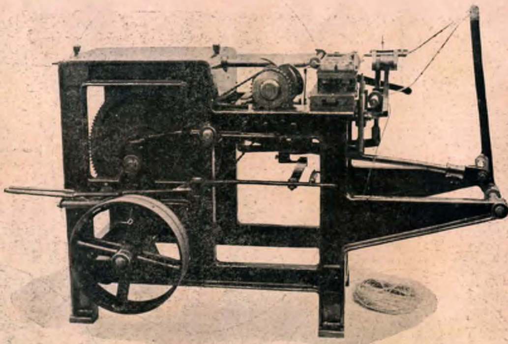
PATENTES NÚMS. 102, 347 Y 30.137 COSEDORA LATERAL PARA SUELAS DE ALPARGATAS
