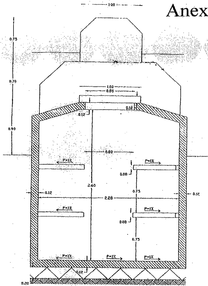
DETALLE TIPO DE PANTEON E:1/20
