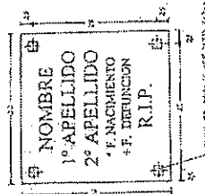
DETALLE DE LAPIDA
